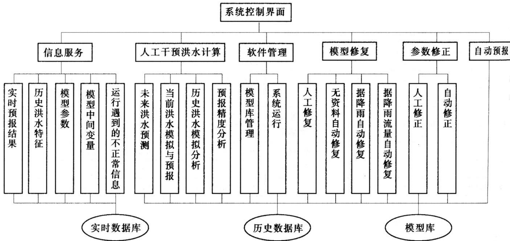
洪水预报系统模块图
